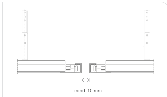
DEHNUNGSFUGE
