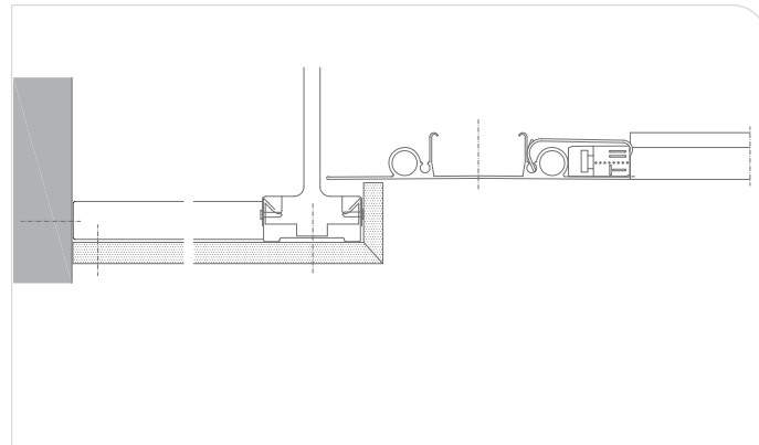
WANDANSCHLUSS GK FRIES
