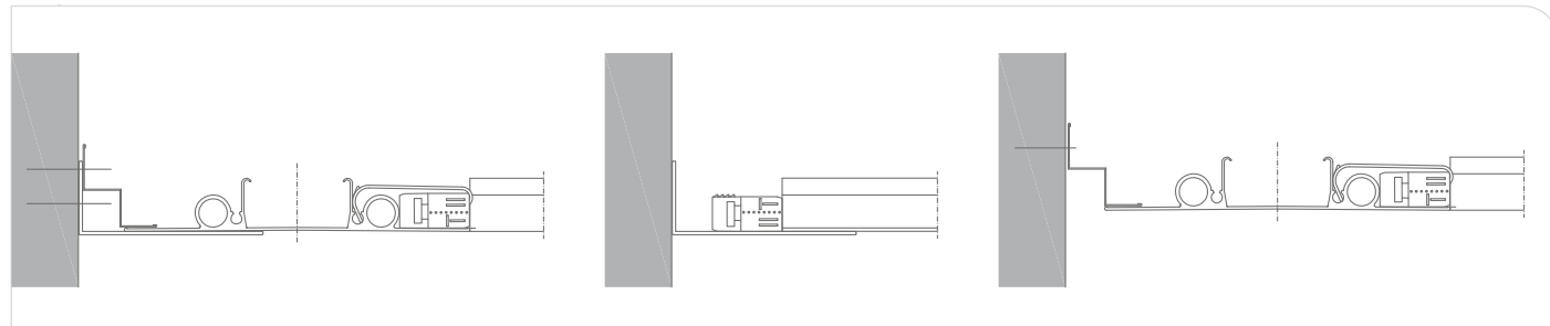
DEHNUNGSFUGE
